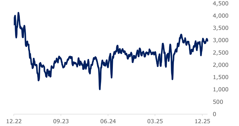
PTF (7 Günlük Ortalama, TL/MWh)
